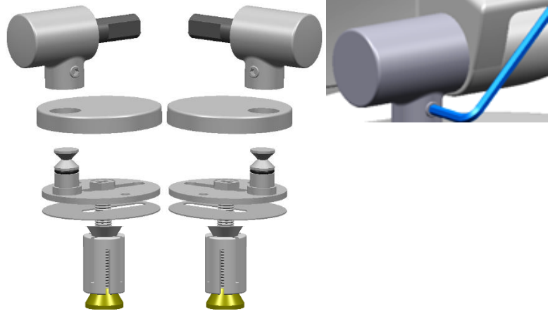
Scharnier
