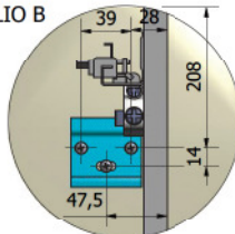
DETTAGLIO B
