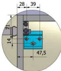
DETTAGLIO A
